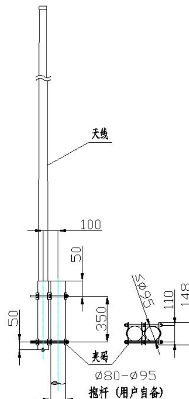
安装示意图
